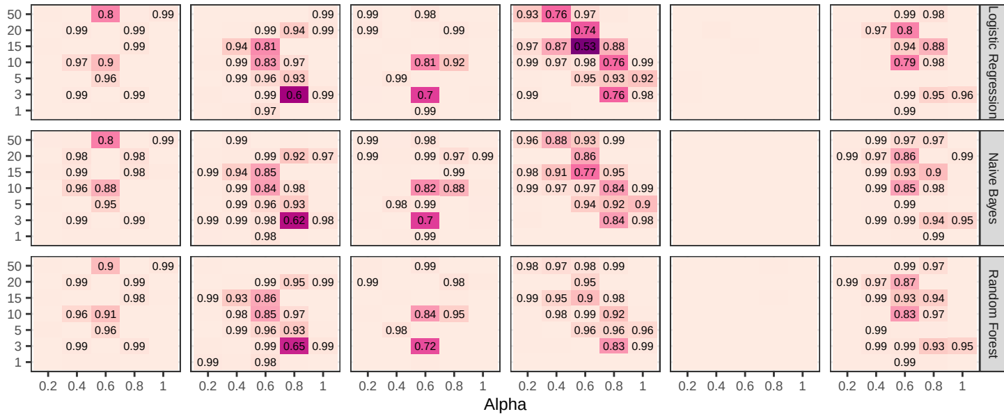
Wikitext
