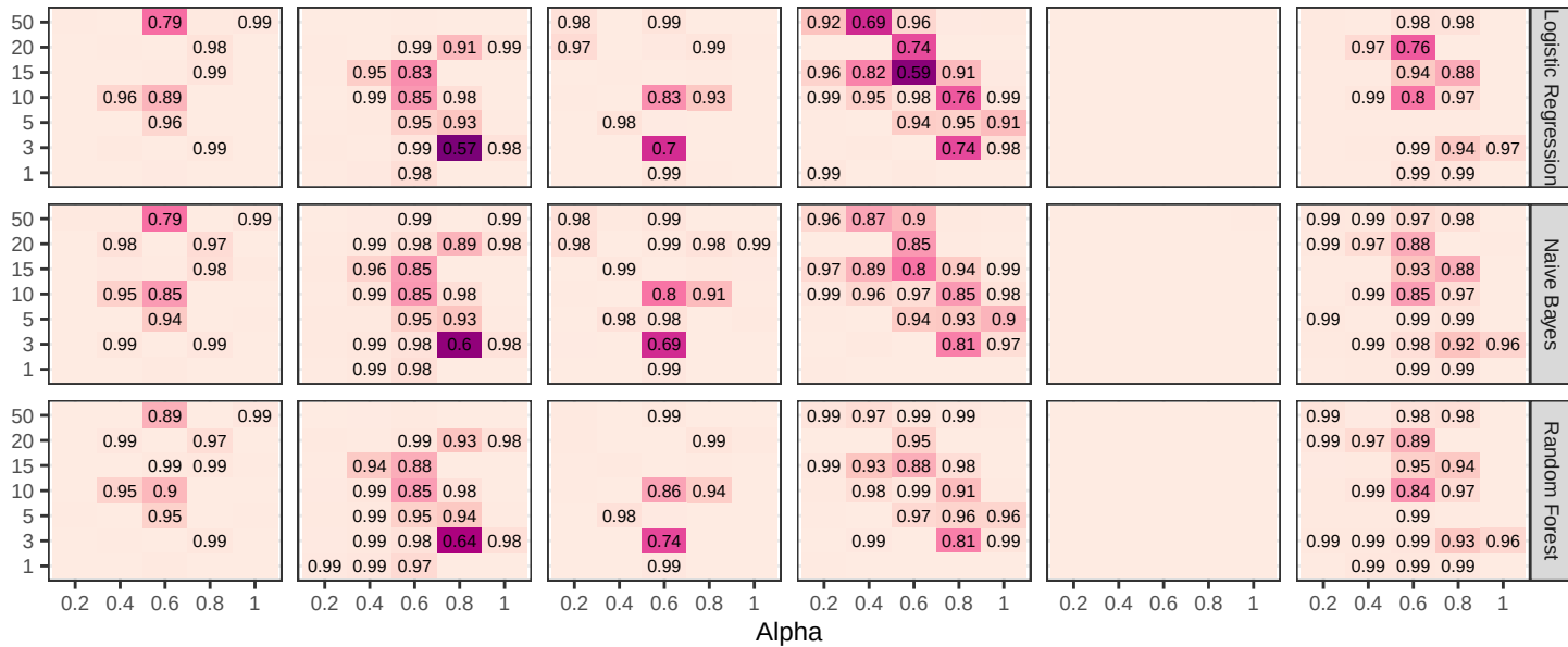
Wiktext
