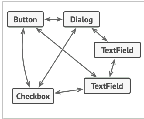
Login Dialog
