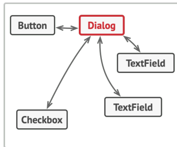
LogIn Dialog
