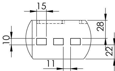
DETALLE A
