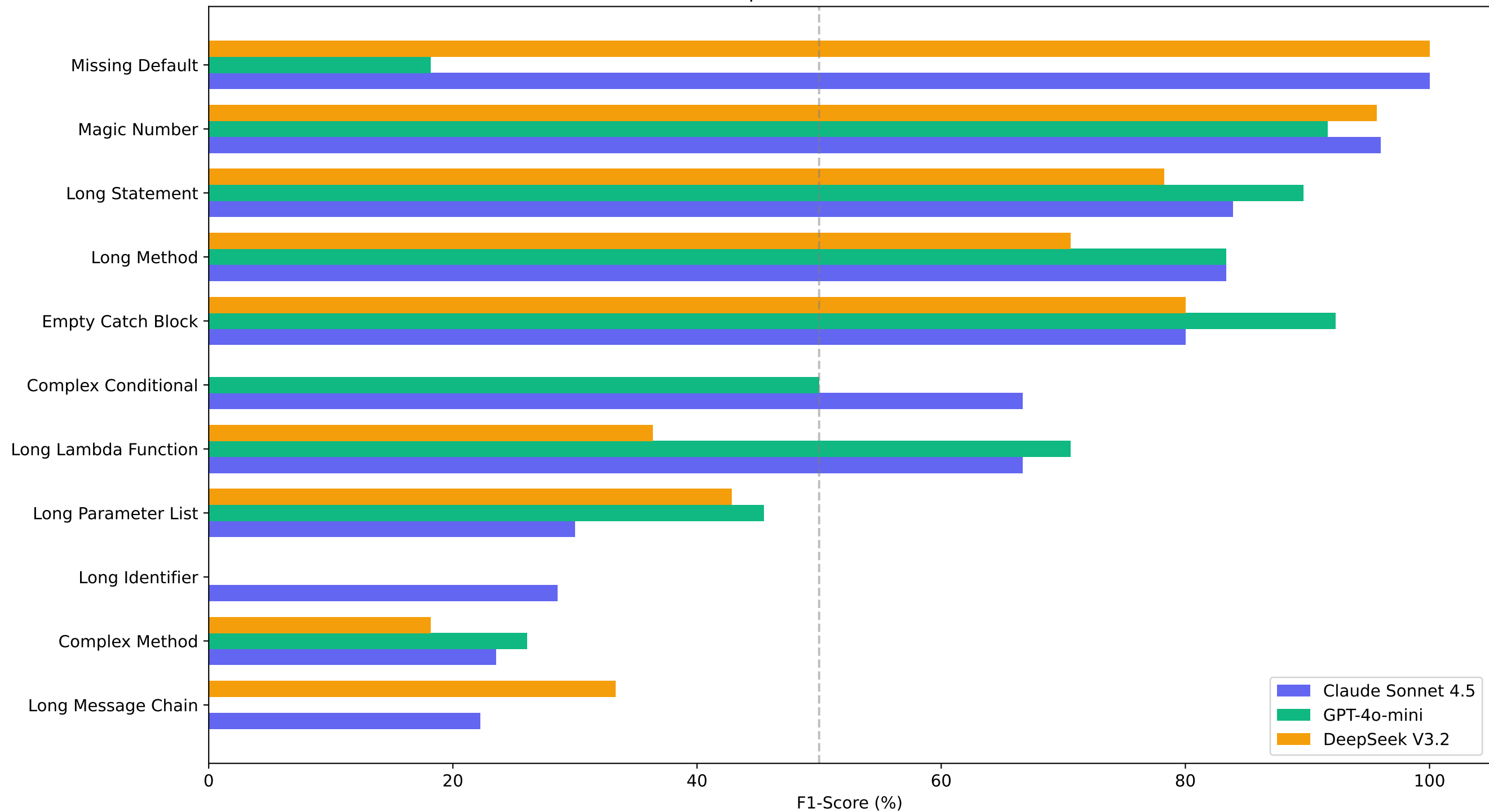
F1-Score por Code Smell e Modelo LLM
