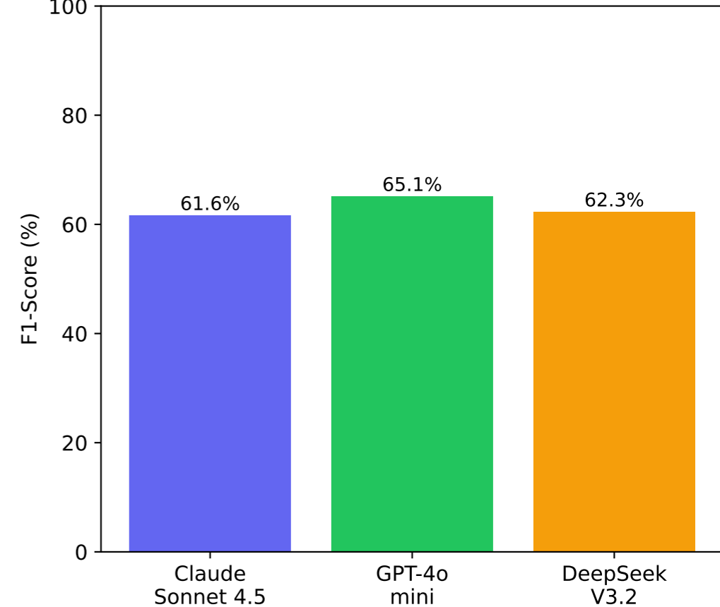
Qualidade (F1)
