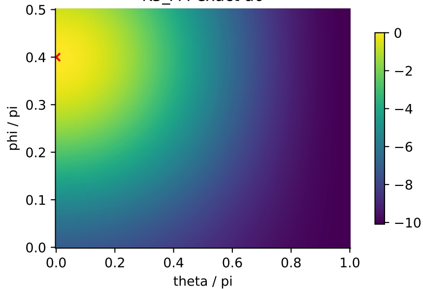
K5_A : exact a0
