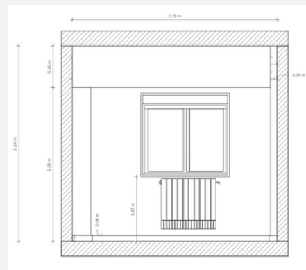
Alzados, secciones y detalles de instalación
