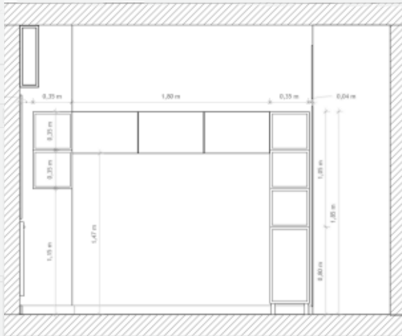
Planos de instalación
