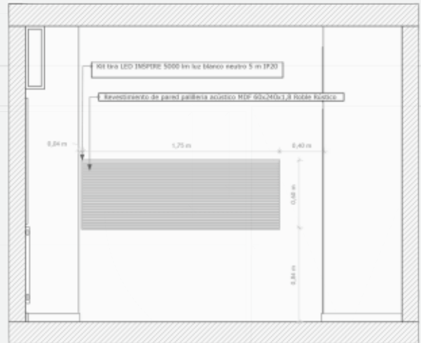
Planos de instalación
