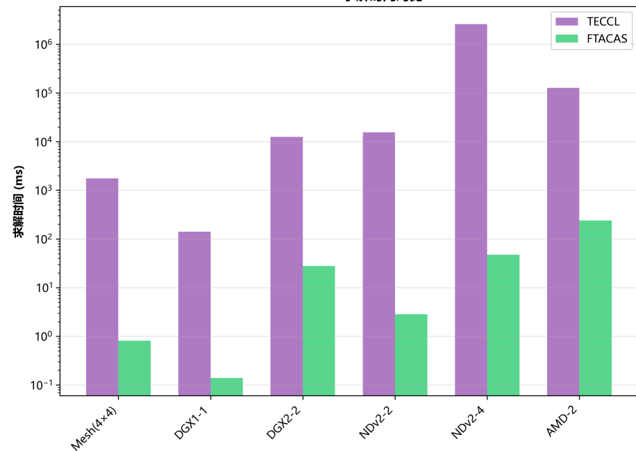
AllToAll 求解时间对比
