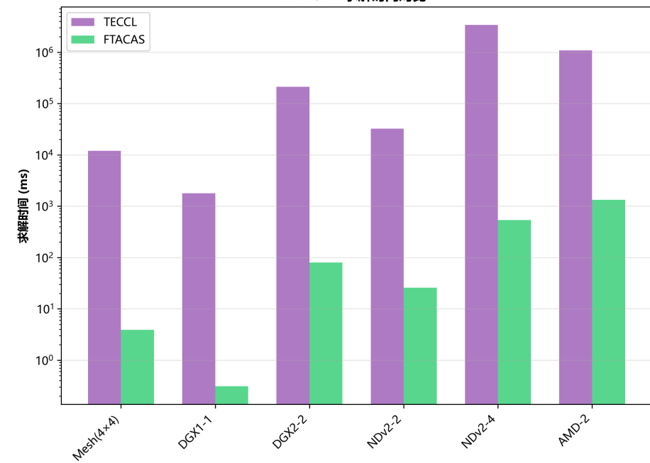
AllToAll 求解时间对比
