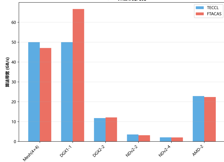
AllToAll 算法带宽对比
