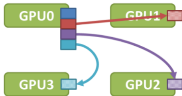
Scatter
