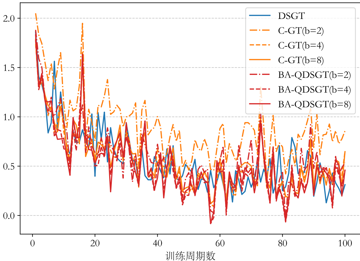
损失函数值
