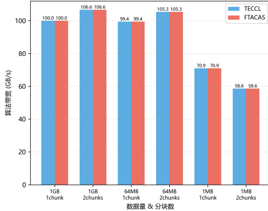
DGX2-2
