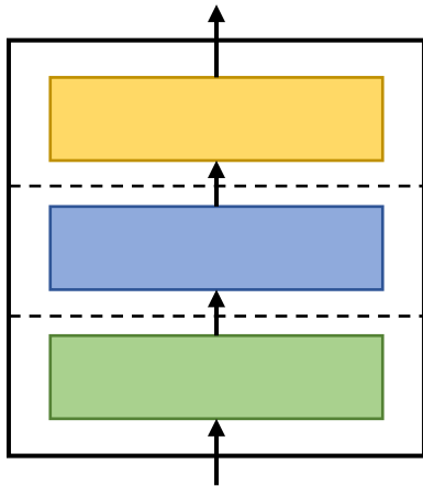
流水并行
