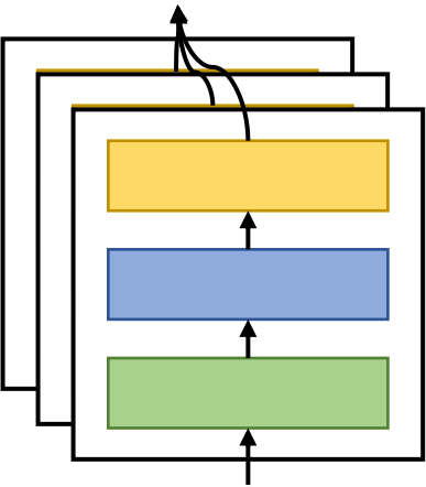
数据并行
