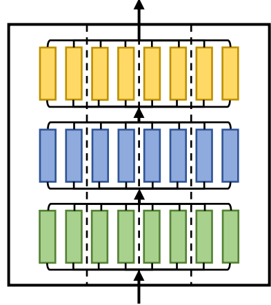
专家并行
