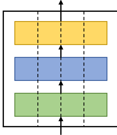
张量并行
