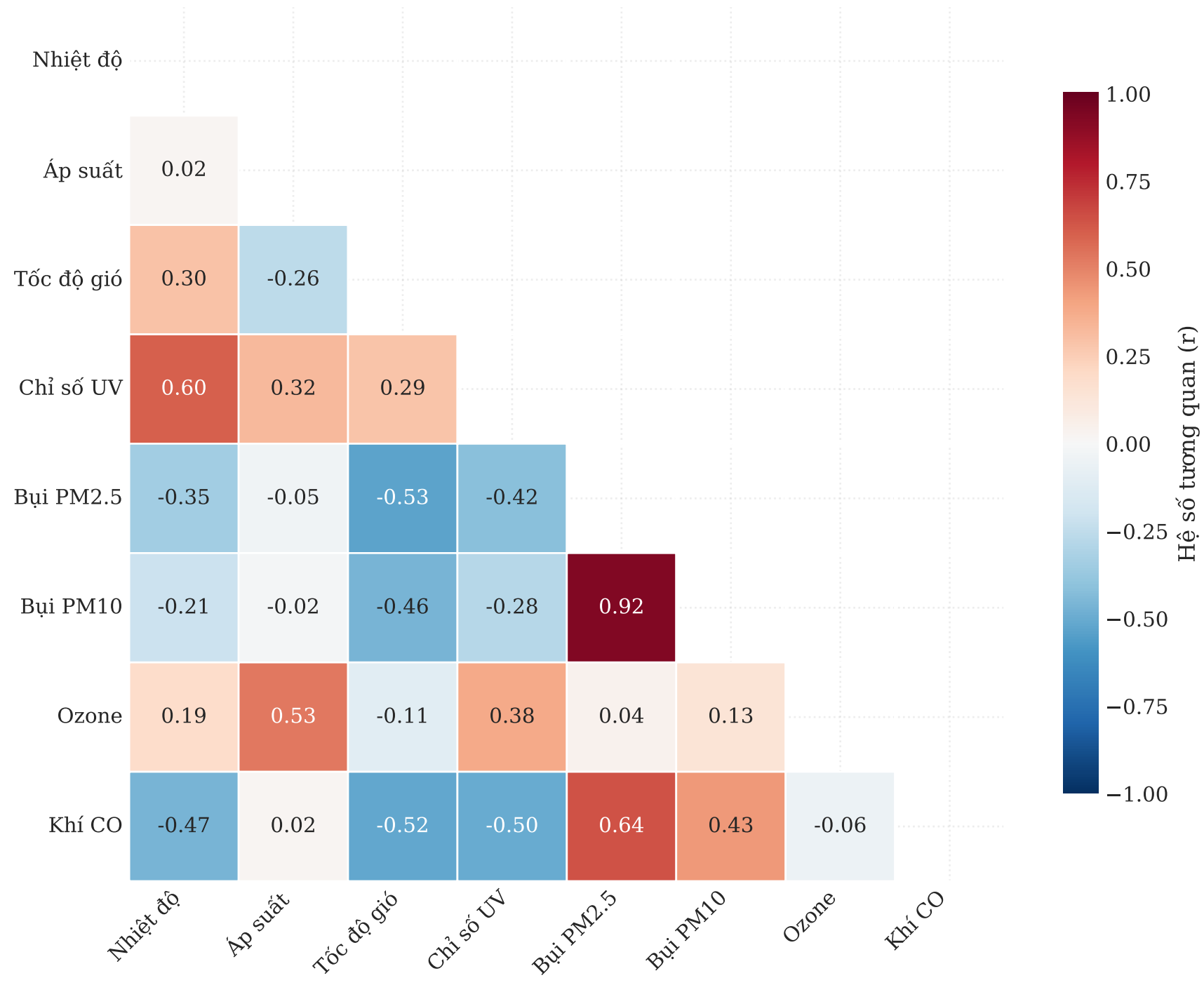
HÌNH 5: Ma trận tương quan (TP.HCM 2024)
