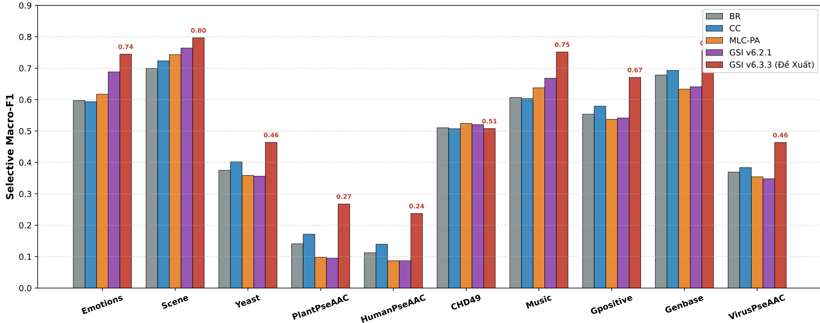
ĐỐI SÁNH SELECTIVE MACRO-F1 TRÊN 10 TẬP DỮ LIỆU BENCHMARK (LOGISTIC REGRESSION BASE LEARNER)
