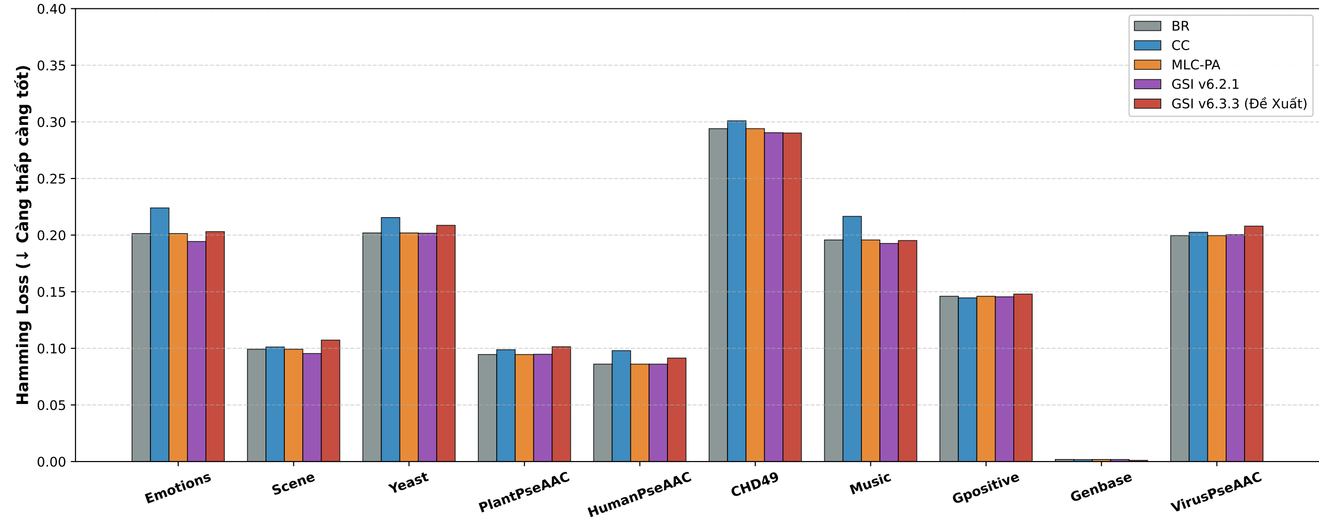
Đối Sánh Hamming Loss Trên 10 Tập Dữ Liệu (Sai Số Bit Từng Nhãn)
