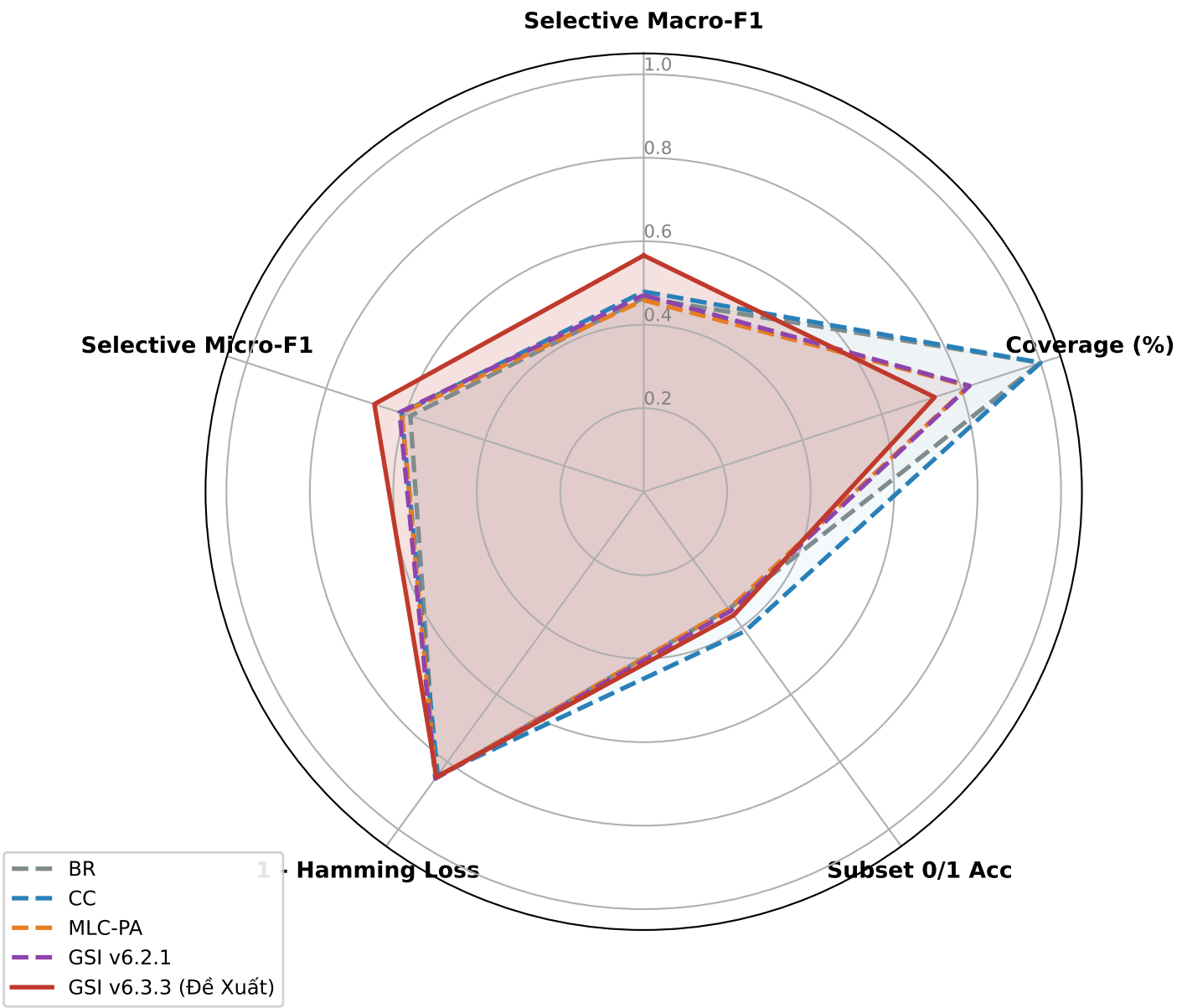
Biểu Đồ Radar Đối So Sánh Đa Mục Tiêu Giữa 5 Hệ Thống Mô Hình
