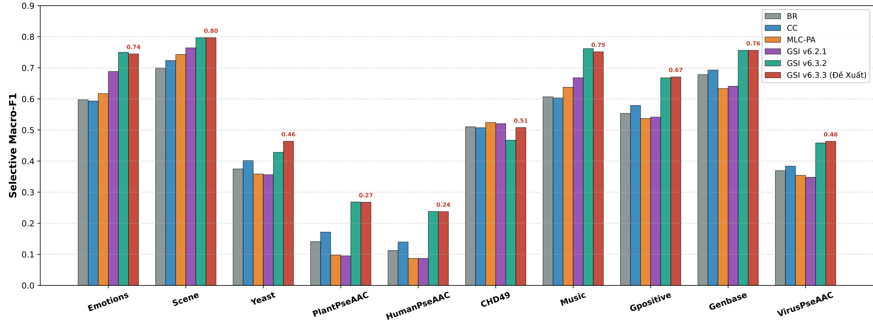
ĐỐI SÁNH Selective Macro-F1 TRÊN 10 TẬP DỮ LIỆU BENCHMARK (LOGISTIC REGRESSION BASE LEARNER)
