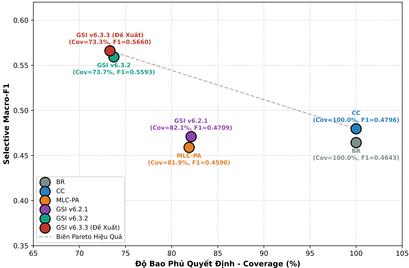
Đồ Thị Đánh Đổi Pareto Giữa Độ Phủ Quyết Định và Selective Macro-F1
