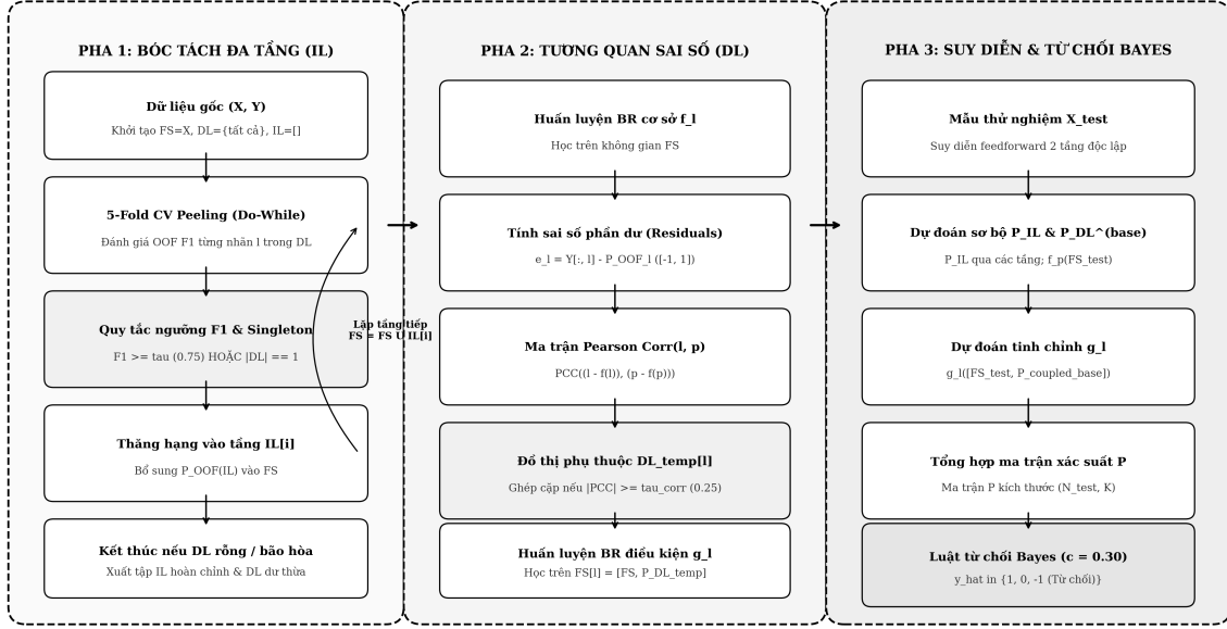
Hình 1: Sơ đồ luồng xử lý 3 giai đoạn của mô hình GSI-MLC-PA v6.2.1. Giai đoạn 1 bóc tách nhân độc lập (IL) với cơ chế hạ ngưỡng đa tầng \tau_{\text{stage}} \in \{0.75, 0.70, 0.65\} . Giai đoạn 2 ước lượng xác suất ngoại mẫu (OOF), tính sai số phần dư e_l , xây dựng ma trận tương quan sai số Pearson để khám phá đồ thị có hướng thừa G_{DL} và chỉ huấn luyện chuỗi mở rộng cục bộ trên các nhân phụ thuộc. Giai đoạn 3 áp dụng luật quyết định Bayes với chi phí từ chối cố định c = 0.30 .
