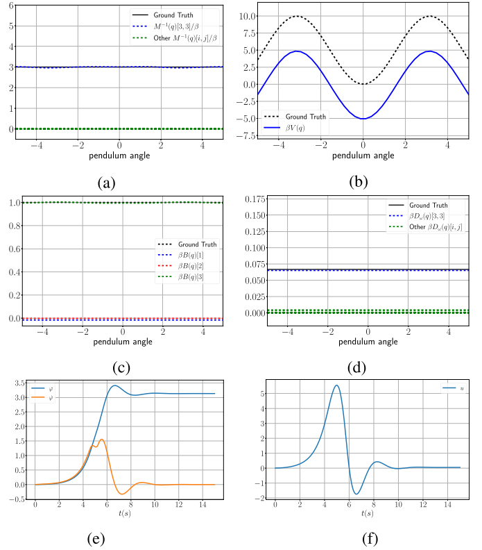
图3. 使用具有尺度因子 \beta = 1.33 的 SO(3) port-Hamiltonian 神经 ODE 网络进行摆的动力学估计。(a) \mathbf{M}^{-1}(\mathbf{q})/\beta 对 \varphi 。(b) \beta \mathcal{V}(\mathbf{q}) 对 \varphi 。(c) \beta \mathbf{B}(\mathbf{q}) 对 \varphi 。(d) \beta \mathbf{D}_{\omega}(\mathbf{q}) 对 \varphi 。(e) 角度 \varphi 和速度 \dot{\varphi} 。(f) 控制输入 u 。
