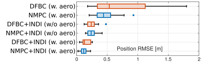
图1: 上: 我们的四旋翼无人机跟踪赛道轨迹。下: 箱线图比较了NMPC、DFBC及其带有INDI内环的变体的位置信息跟踪均方根误差 (RMSE), 并区分是否考虑空气动力阻力效应。对于每种方法, 数据均来自实际飞行, 跟踪不同参考轨迹, 其速度高达 20 m/s (即72 km/h), 加速度高达5g。
