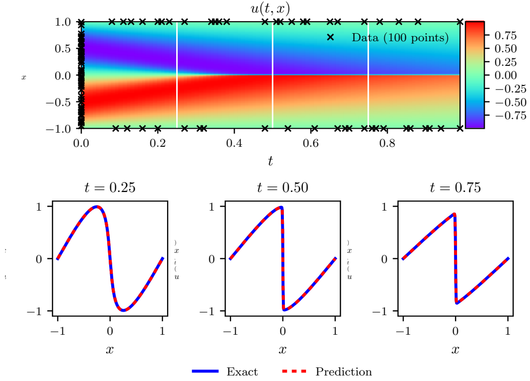
图 1: Burgers' equation : Top: 预测解 u(t, x) 以及初始和边界训练数据。此外，我们使用拉丁超立方抽样策略生成了 10,000 个配点。Bottom: 对应顶面中白色垂直线描绘的三个时间快照，预测解和精确解的比较。该情况下的相对 \mathcal{L}_2 误差为 6.7 \cdot 10^{-4} 。模型训练在单个 NVIDIA Titan X GPU 上大约耗时 60 秒。
