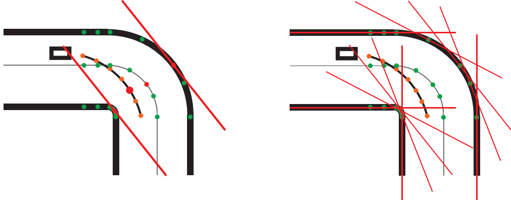
图4: 左: 水平线上某一点(大红点)的半空间约束(红线)。右: 整个水平线的生成半空间(红线), 近似轨迹。中心线上绿色的点对应于水平线上每个点在离散中心线上最近的点。边界上的点是中心线点在边界上的投影。
