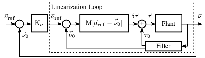
图3: 基于INDI的速度控制器框图
