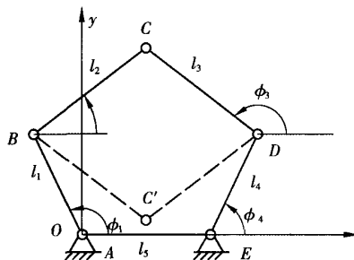
图1 平面五杆机构运动学分析简图
