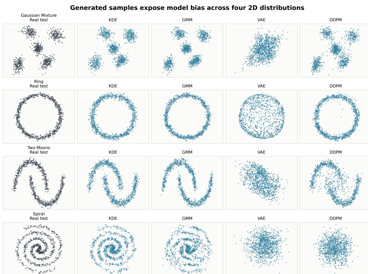
图 2: 四类模型在四类二维分布上的生成样本。灰色点为测试样本，蓝色点为生成样本。KDE/GMM 在低维任务中非常强；VAE 明显过平滑；DDPM 长训练后在 Spiral 上能更好跟随螺旋支撑。
