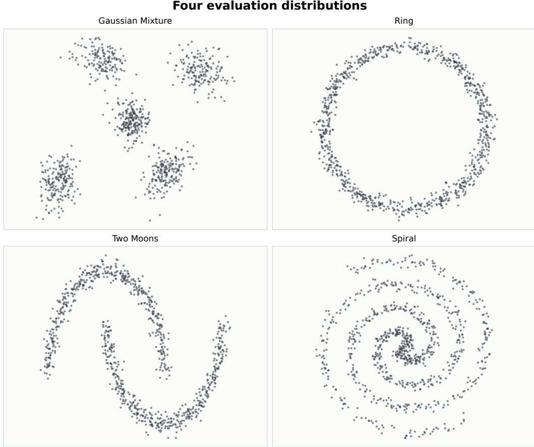
图 1: 四类二维测试分布。Gaussian Mixture 呈现离散多峰结构；Ring 具有中心空洞；Two Moons 是两个弯曲月牙；Spiral 具有长程螺旋支撑。
