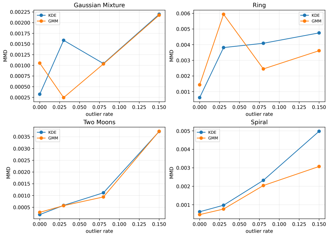
图 5: 向训练集中加入不同比例均匀异常点后, KDE 和 GMM 的 MMD 变化。
