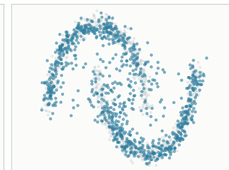
DDPM
