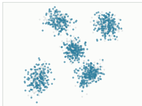
KDE
