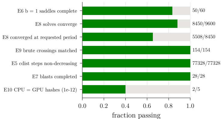
(d) robustness scorecard
