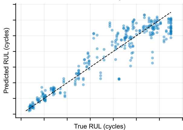
FD003: GRU window50
