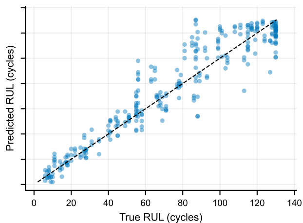
FD003: GRU window50
