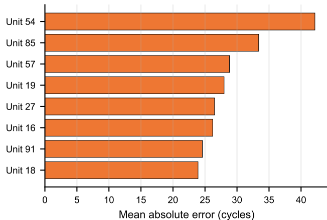
FD003: GRU window50
