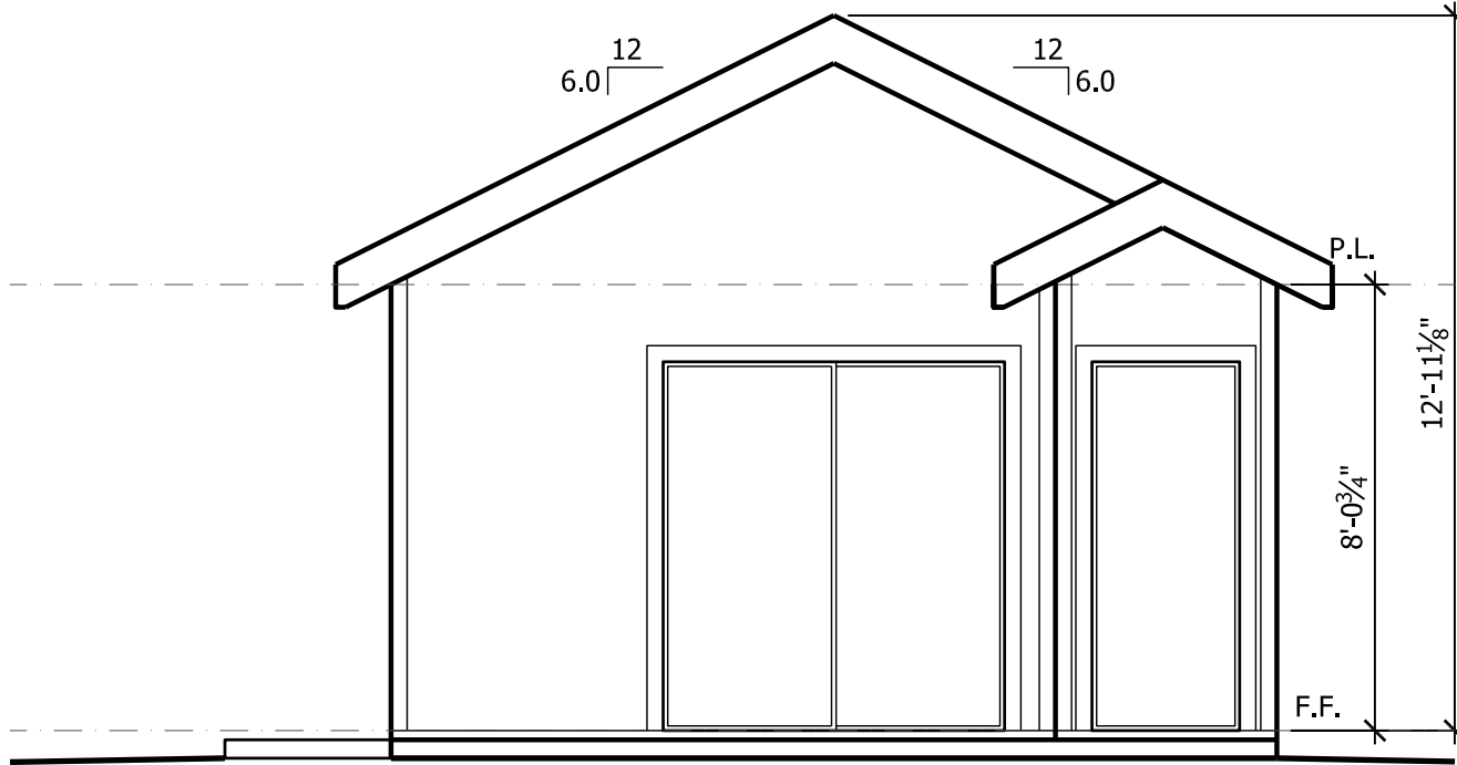
B RIGHT ELEVATION
