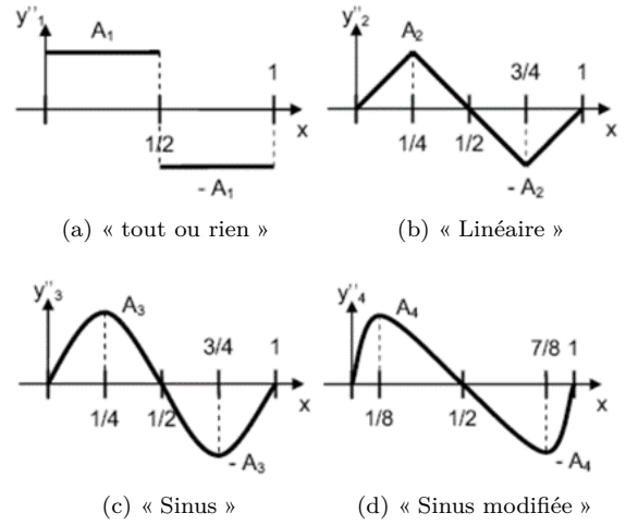
FIG. 4 – Lois d'accélération en coordonnées réduites y''(x)
