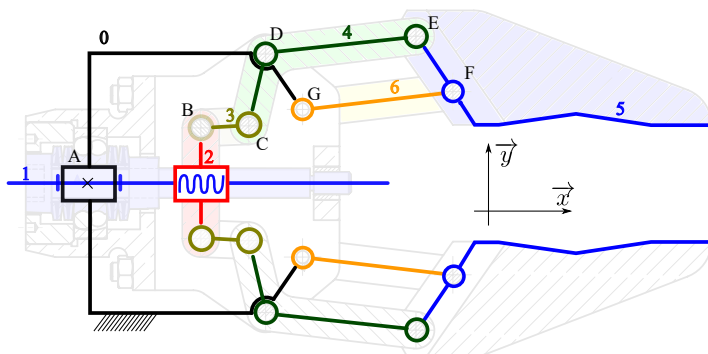
FIG. 4 – Schéma cinématique
