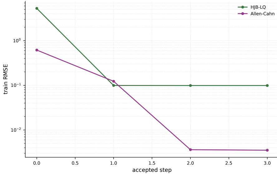
图 3.1 半线性方程的 LM 迭代残差下降
