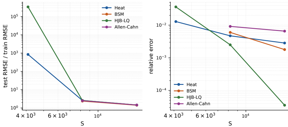
图 4.2 样本数对泛化比值和初值相对误差的影响
