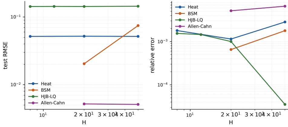
图 4.3 随机特征宽度对测试残差和初值相对误差的影响
