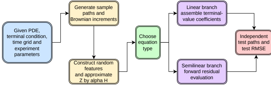
图 3.1 实验求解方法的整体流程
