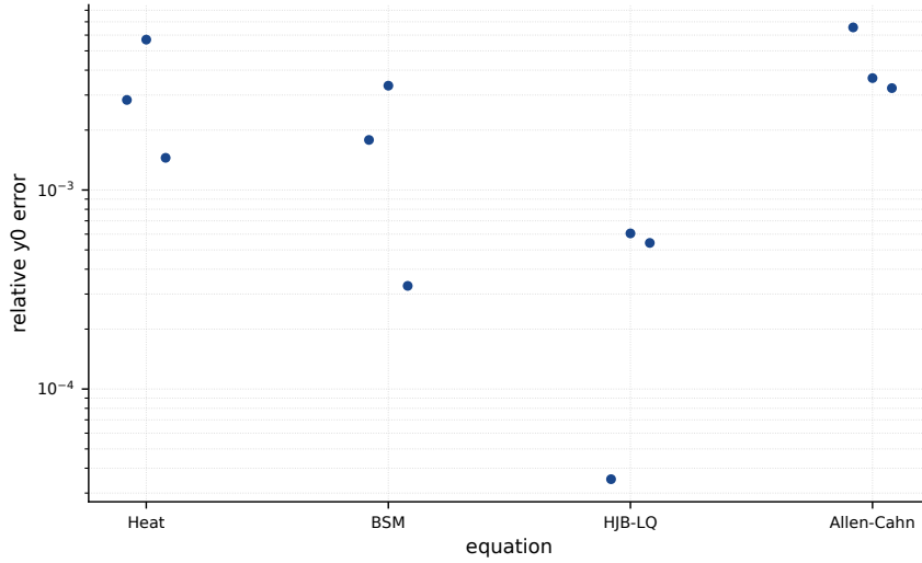
图 4.5 不同随机种子下的初值相对误差
