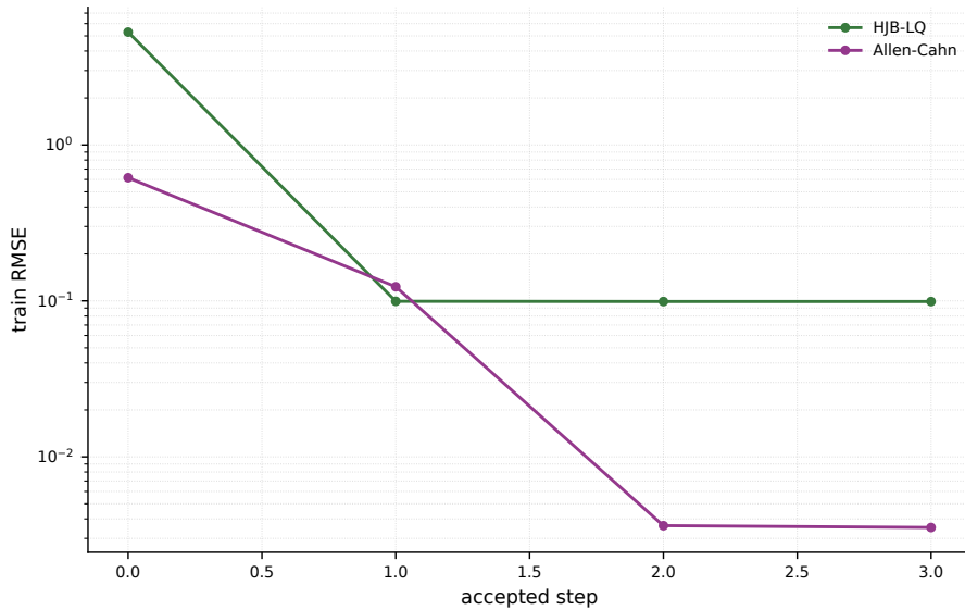
图 4.1 半线性方程的 LM 迭代残差下降
