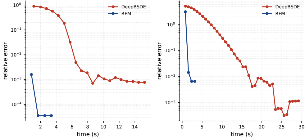
图 4.6 RFM 与 DeepBSDE 的初值相对误差对比
