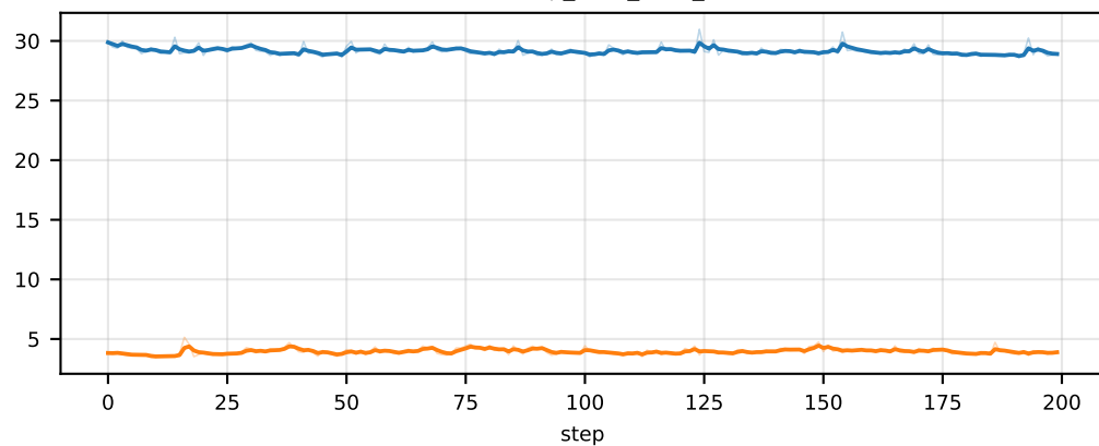
time/ref_log_probs_values_reward
