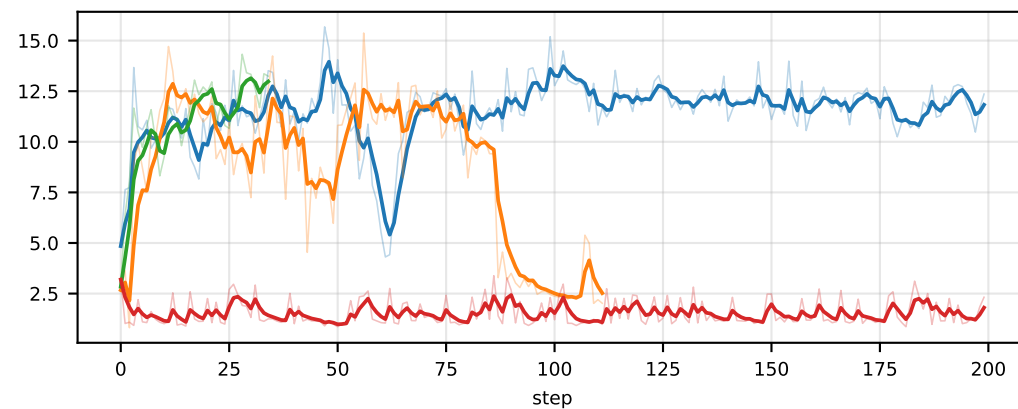
time/old_log_probs_values
