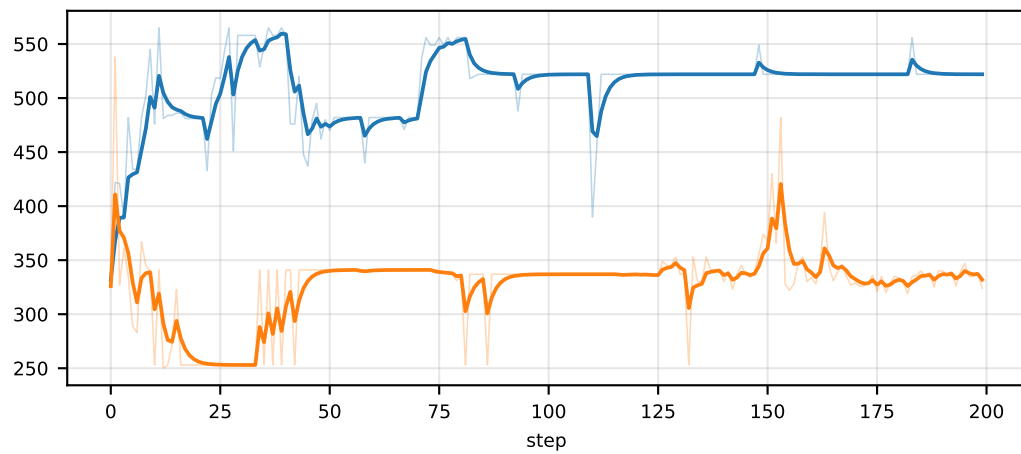
tokens/non_prompt_length/min
