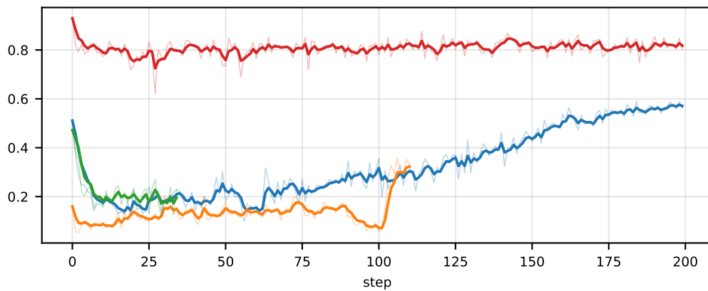
actor/ratio_min
