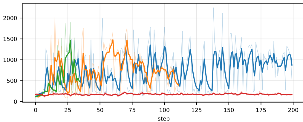
tokens/non_prompt_length/mean
