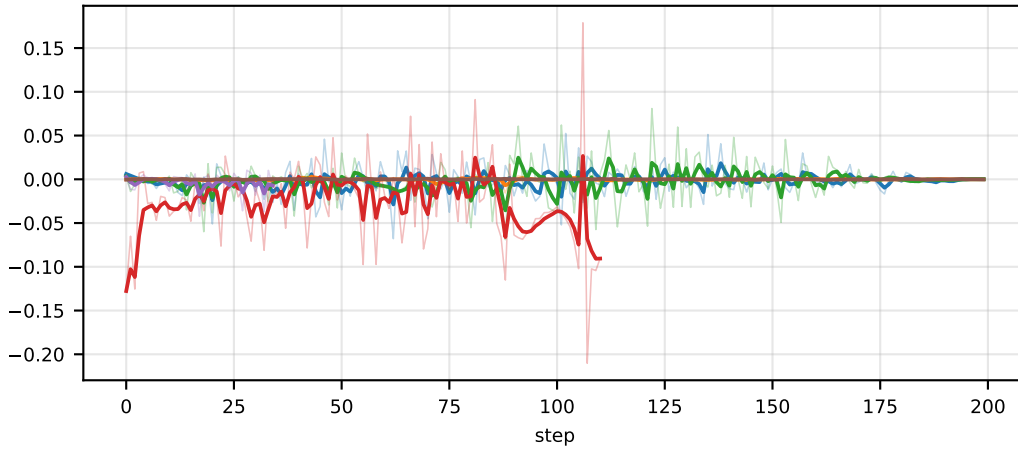
actor/policykl
