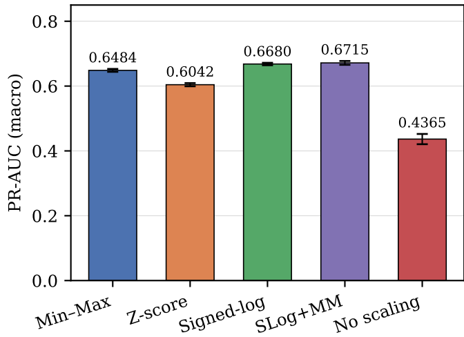
CICIoT2023
