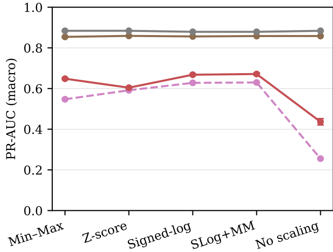
CICIoT2023
