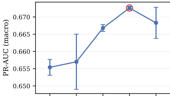
CICIoT2023
