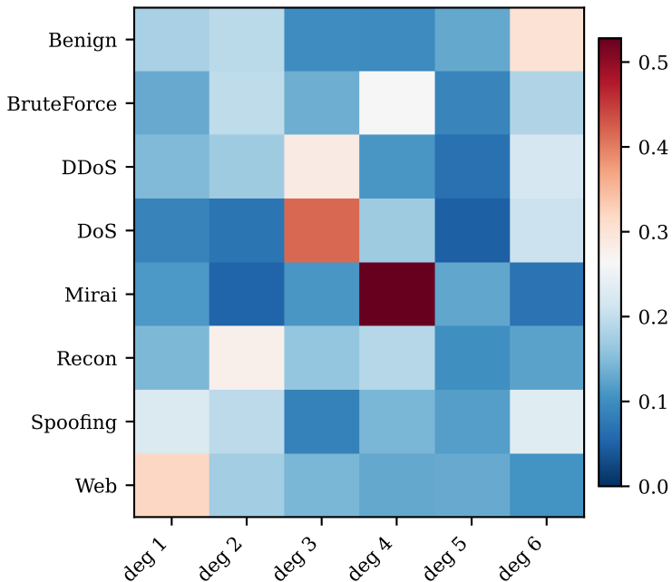
CICIoT2023
