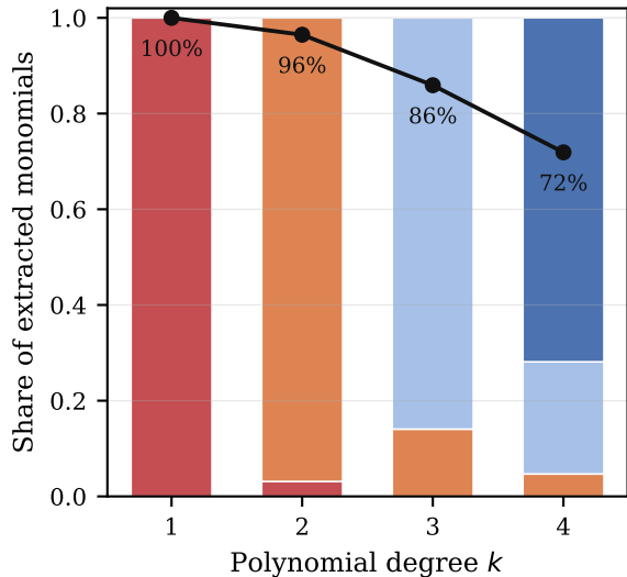
CICIoT2023
