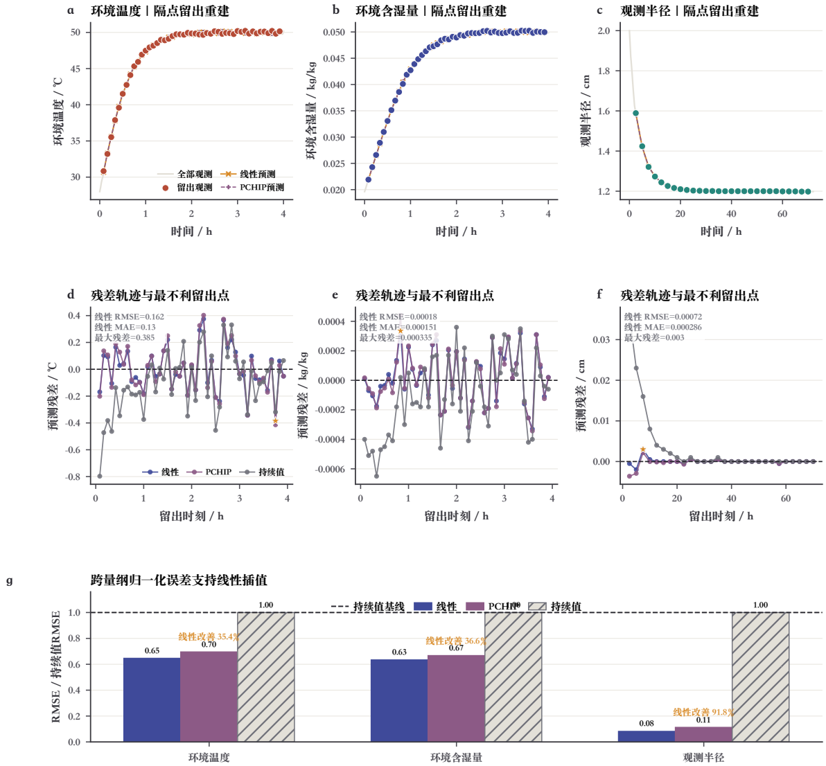
图 10 输入插值留出检验
