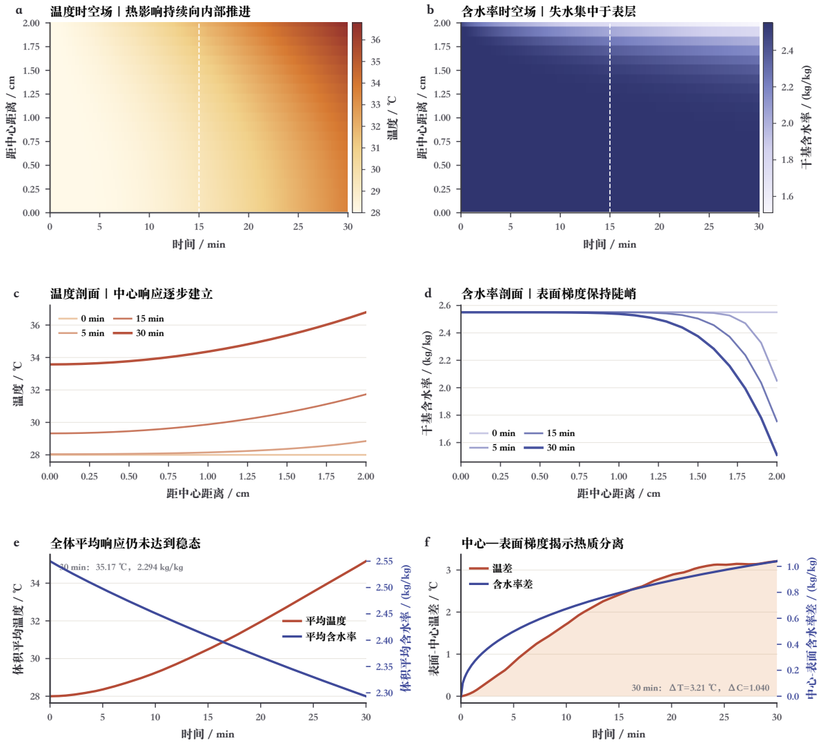
图 4 问题一温湿场演化
