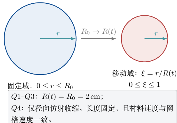
(b) 径向模型与收缩坐标
