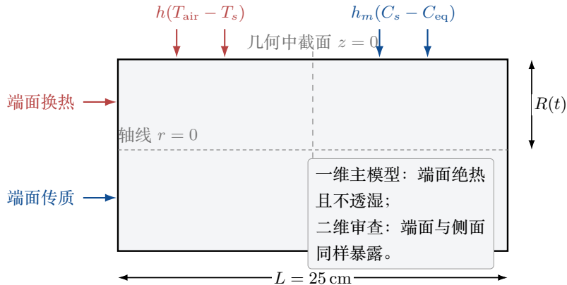
(a) 圆柱几何与端面口径
