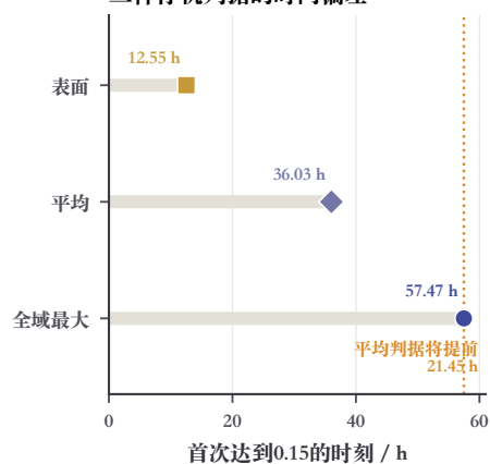
b 三种停机判据的时间偏差
