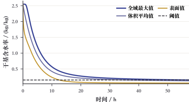
c 判据量的长期分离
