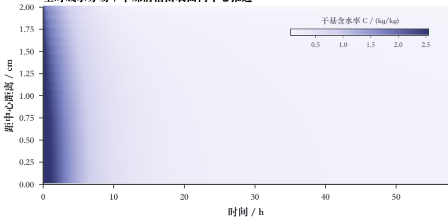
a 全时域水分场 | 干燥前沿由表面向中心推进
