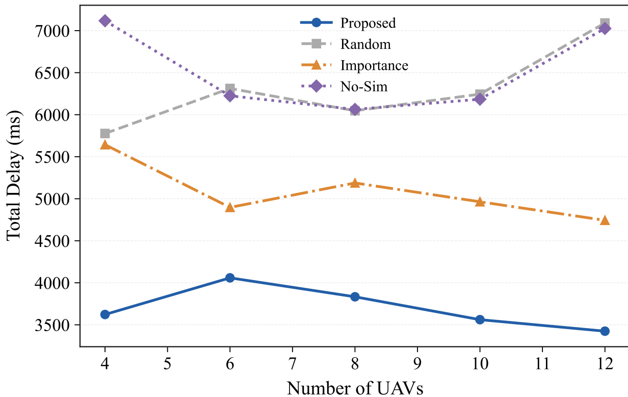
Fig. 7 Real MoE: UAV Count
