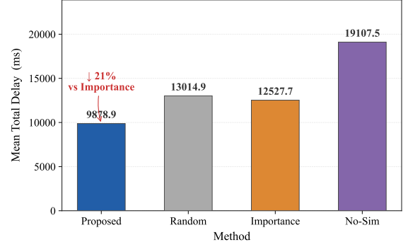
Fig. 3. 不同专家部署方法的平均端到端延迟对比。
