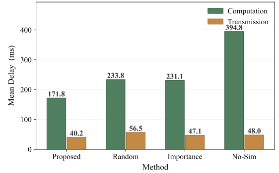
Fig. 4. 端到端延迟分解。SimAeroMoE 通过通信感知部署和逐层调度同时降低计算与传输开销。
