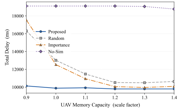
Fig. 8. UAV 内存容量对端到端延迟和部署规模的影响。
