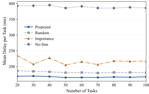
Fig. 10. 任务数量变化下的延迟和规划时间。
