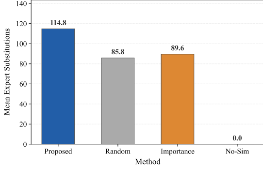
Fig. 5. 相似专家替代次数。Proposed 更充分地利用相似专家覆盖原始专家需求。
