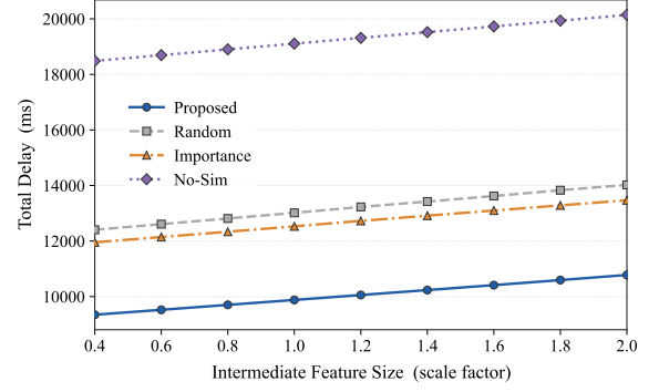
Fig. 7. 中间特征大小对端到端延迟的影响。
