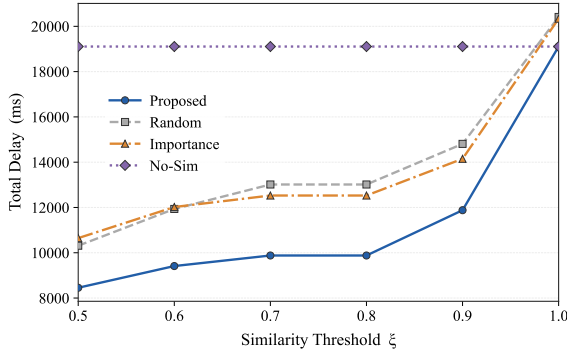
Fig. 6. 相似度阈值 \xi 的敏感性分析。
