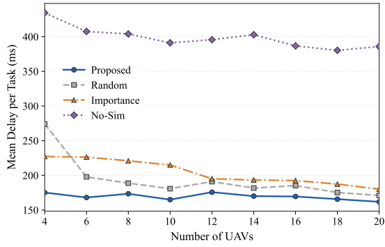
Fig. 9. UAV 数量变化下的扩展性。
