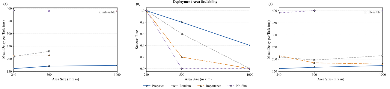
Fig. 12. 部署区域大小变化下的扩展性。固定资源时，大范围场景会因单跳连通性和UAV 内存限制而降低可行性；同步扩展资源后可维持稳定服务。
