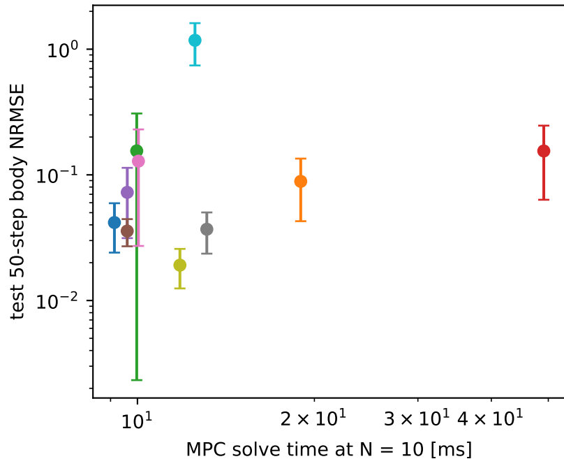
N = 1000 trajectories
