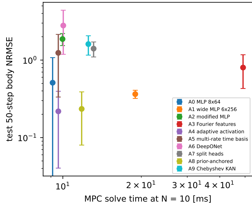
N = 100 trajectories
