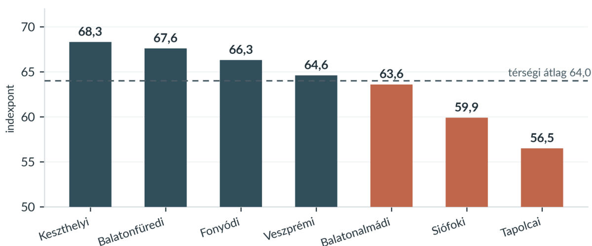
10. ábra. A Balaton Jó Hely Index járásonként, 2026. Sötét: a térségi átlag fölött; terrakotta: alatta.
