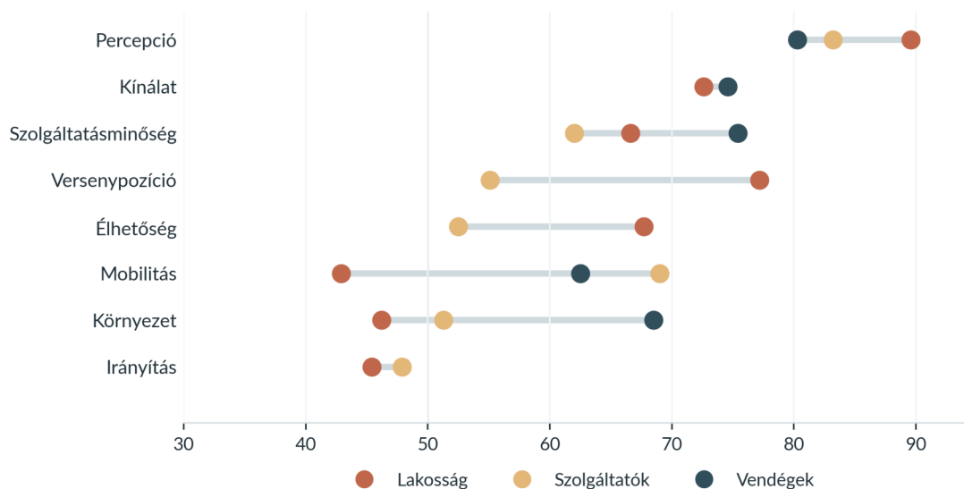
3. ábra. Az alindexek értéke szereplőcsoportonként, 2026.
