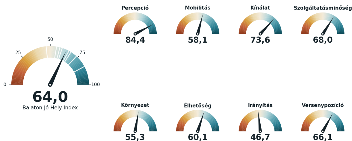
5.2. ábra. A Balaton Jó Hely Index és a nyolc alindex a 0–100 skálán, 2026. A nagy mérőórán a fehér osztások a nyolc alindex helyét jelölik, amelyek 46,7 és 84,4 pont között szóródnak.
