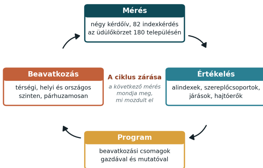
6.3. ábra. A döntési ciklus: a mérés eredménye értékelésen és programon keresztül válik beavatkozássá, a beavatkozás eredményét pedig a következő mérés mutatja meg.
