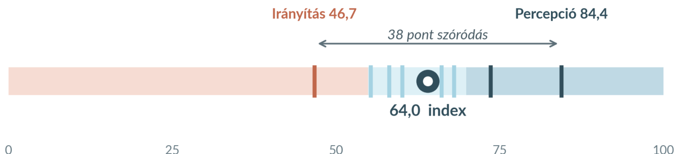
1. ábra. A Balaton Jó Hely Index és a nyolc alindex a 0–100 skálán, 2026. A függőleges osztások az egyes alindexek helyét jelölik.
