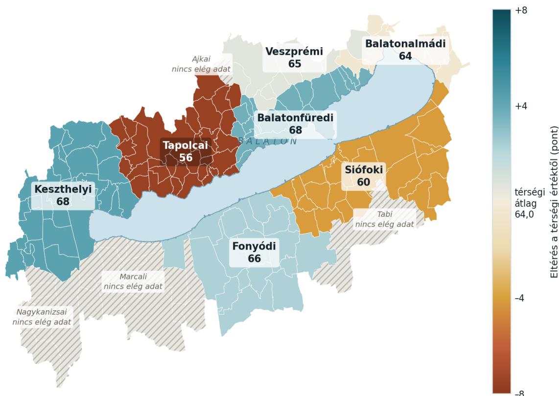
5.7. ábra. A Balaton Jó Hely Index járásonként, 2026. A szín a térségi átlagtól való eltérést mutatja: a kékszöld a fölötte, a terrakotta az alatta lévő járásokat. A vonalkázott járásokban nem volt elég adat az index kiszámításához.
