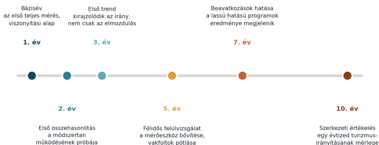
7.3. ábra. A mérés tízéves íve: az idősorból az egyes mérési években levonható következtetések.
