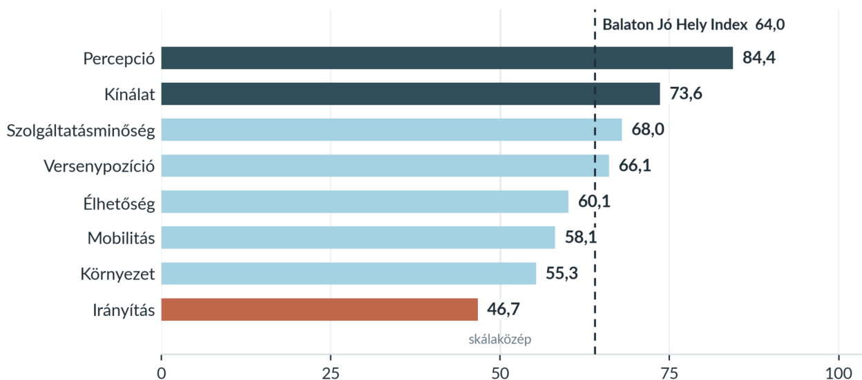
2. ábra. A nyolc alindex értéke, 2026. Sötét: 70 pont fölött; világoskék: 55–70 pont között; terrakotta: 55 pont alatt.
