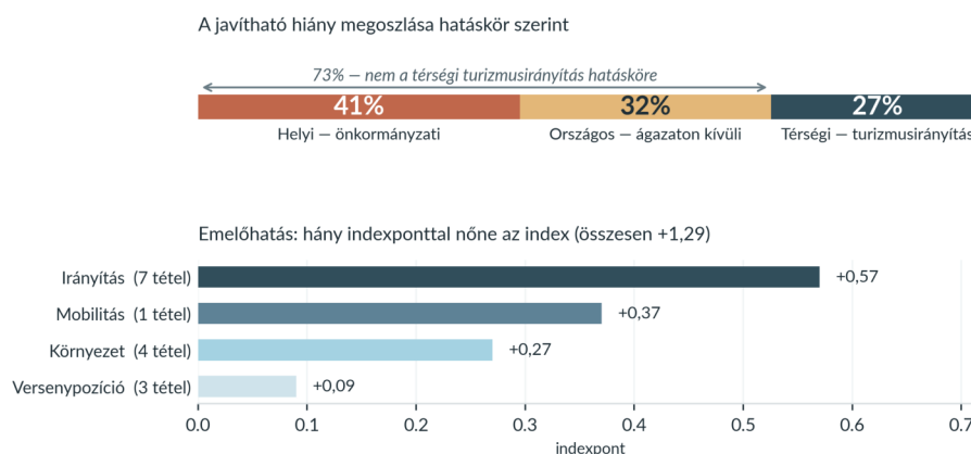
7. ábra. Fent: a javítható hiány megoszlása hatáskör szerint. Lent: hány indexponttal nőne az index, ha az adott alindex skálaközép alatti tételei elérnék az ötven pontot.
