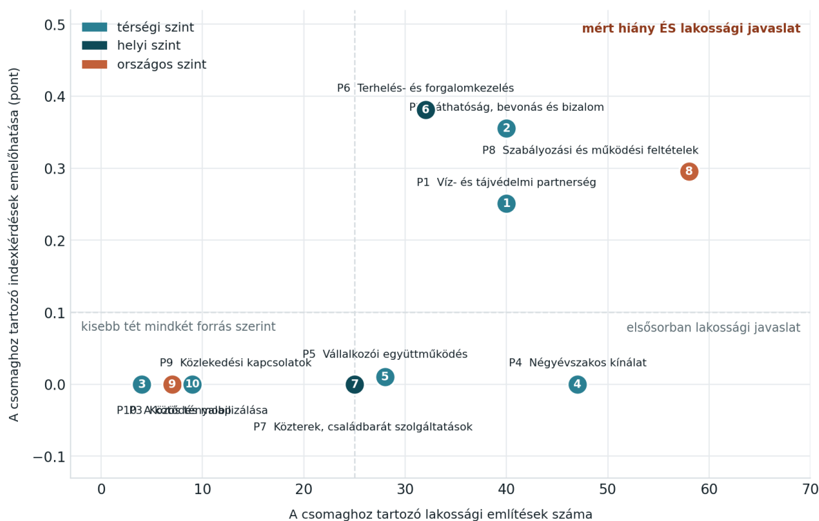
6.5. ábra. A tíz csomag kettős megalapozása: vízszintesen a lakossági említések száma, függőlegesen a csomaghoz tartozó indexkérdések emelőhatása.
