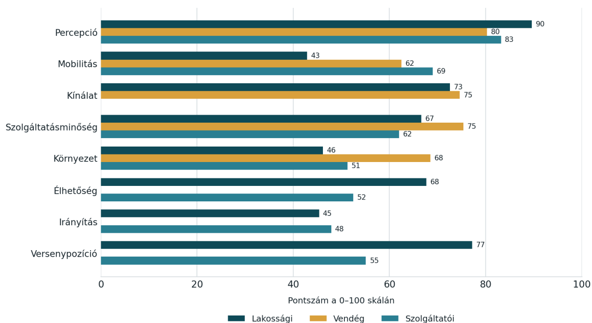
5.4. ábra. Az alindexek értéke szereplőcsoportonként, 2026.
