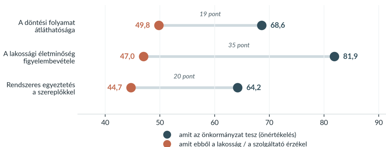
9. ábra. Ugyanaz a téma két nézőpontból: az önkormányzatok önértékelése, illetve a lakosság és a szolgáltatók megítélése.
