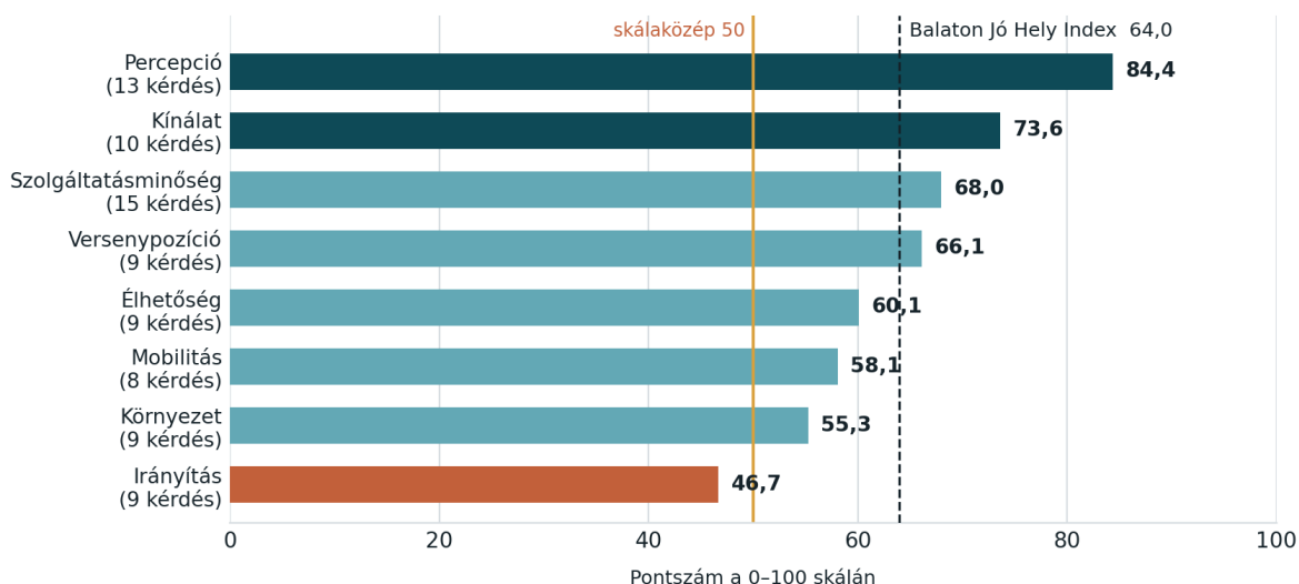
5.3. ábra. A nyolc alindex értéke és a Balaton Jó Hely Index, 2026. A sötét sáv a hetven pont fölötti, a világos az 55–70 pont közötti, a terrakotta az 55 pont alatti alindexeket jelöli.
