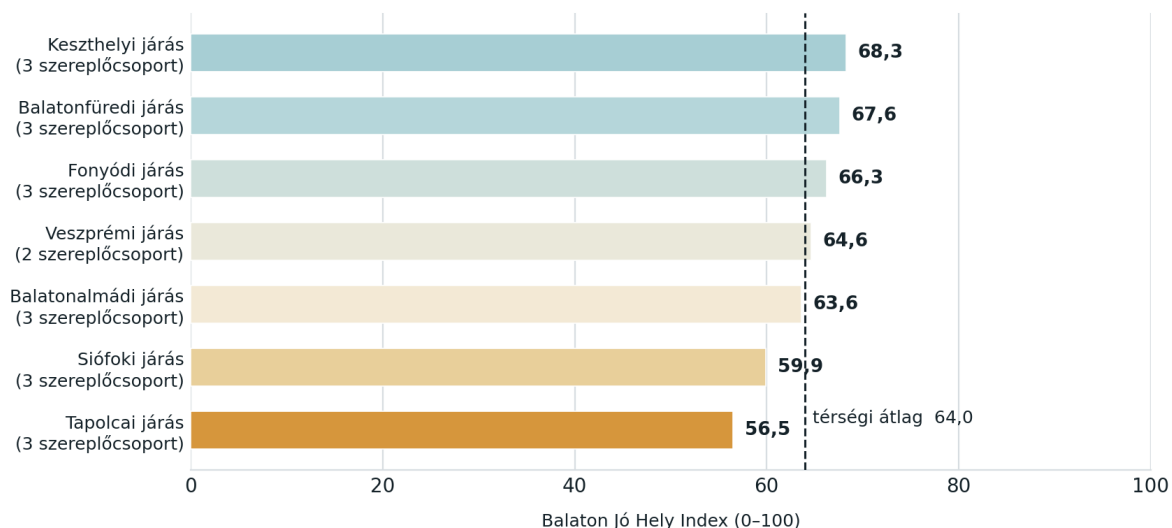
5.8. ábra. Az érvényes indexű járások, 2026.
