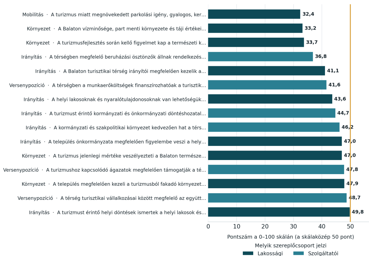
5.5. ábra. A skálaközép alá eső tizenöt kérdés a 82 közül, csökkenő pontszám szerint. A szín azt jelzi, melyik szereplőcsoport adta az értékelést.
