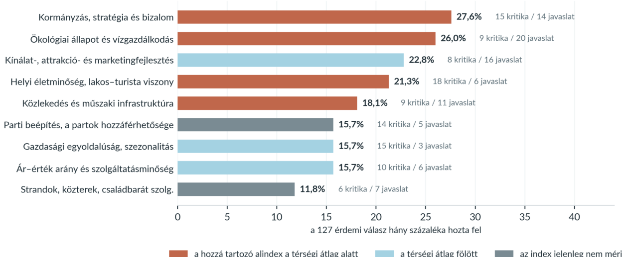
8. ábra. A nyílt kérdés témái említésszám szerint. A szín azt jelzi, hogy a témához tartozó alindex a térségi átlag alatt vagy fölött áll-e.
