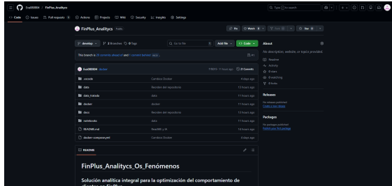
Figura 4: Repositorio GitHub.
