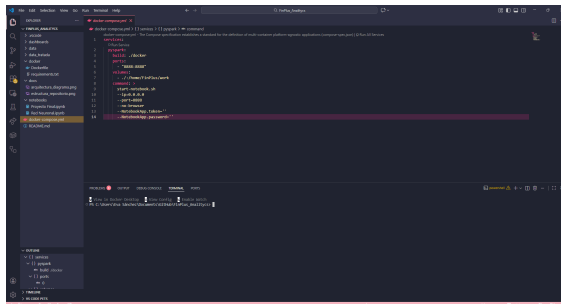
Figura 2: Archivo docker-compose.yml.
