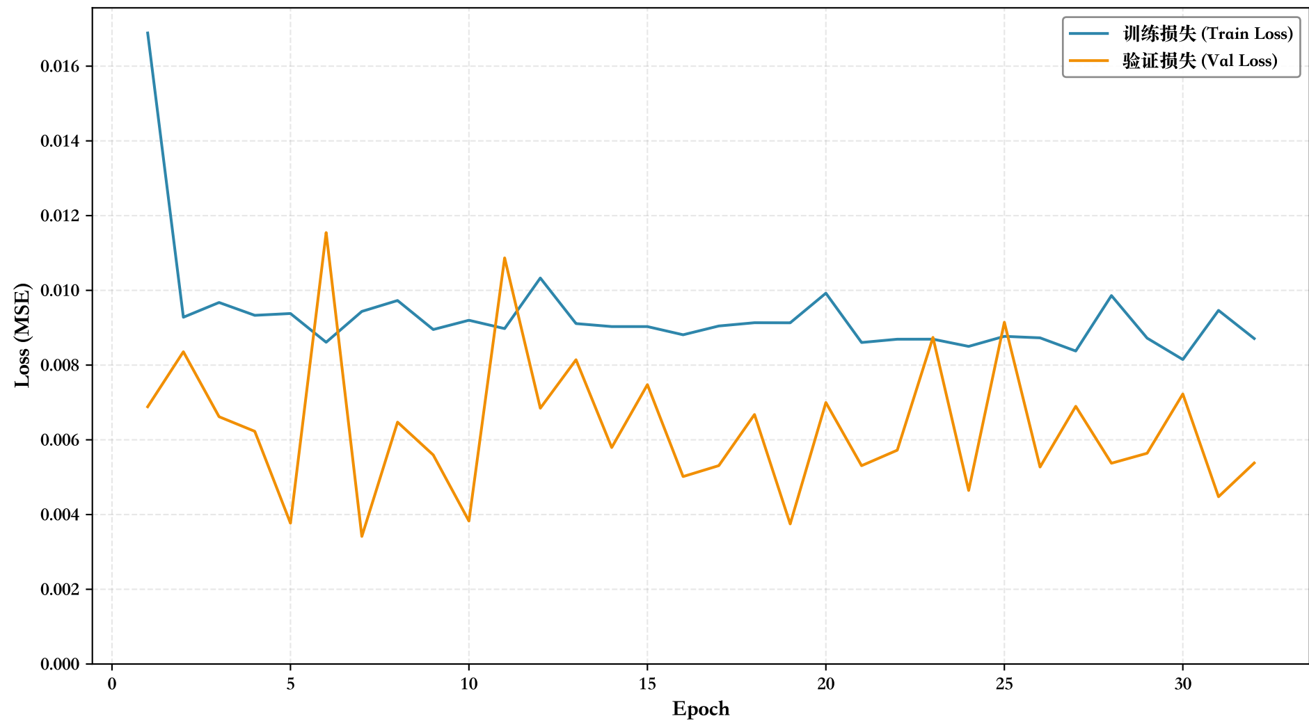
训练/验证损失曲线 - GRU
